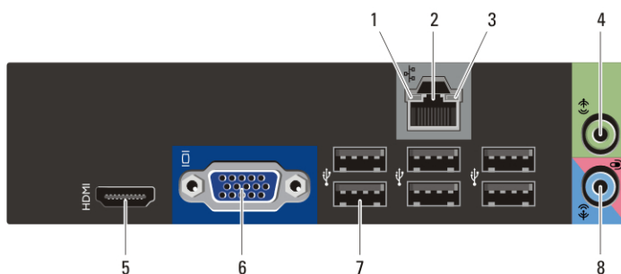
Slika 5. Prikaz zadnjeg panela za Small Form Factor kućište
